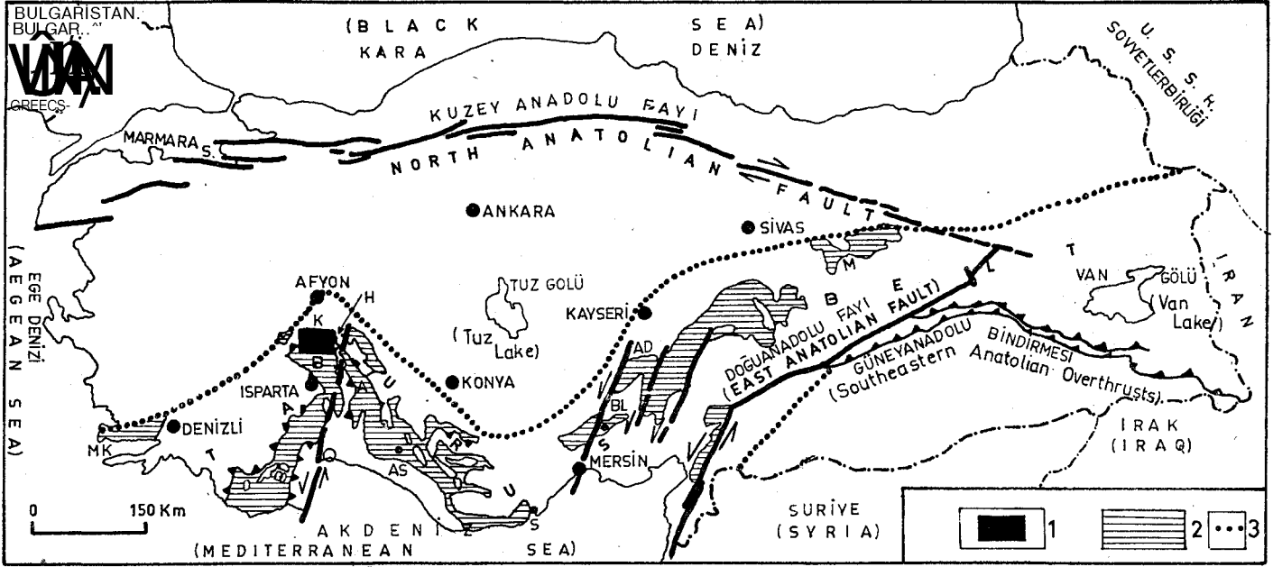
Şekil 1 : Toros Kuşağı yarı otokton platform seâimanlarının dağılımı ve büyük yapısal çizgileri gösterir harita (Adamia ve diğerleri, 1980'den yalınlaştırılmıştır). 1. Çalışma alanı; 2. Toros Kuşağı yarı otokton platform sedimanları; 3. Toros Kuşağı yaklaşık sınırı; A. Ananias Dağları; AD. Aladağlar; AS. Akseki; B. Barladağ; BD. Bçydağları; BL. Beledemedik; H. Hoyran gölü dolay; K. Kılıçlağm Dağı; M. Munzur Dağları; MK. Mandalya Körfezi.
