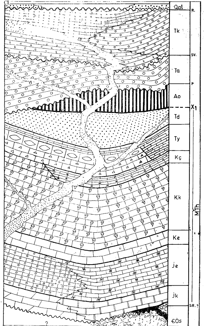
Şekil 2 : İnceleme alanındaki jeoloji birimlerinin stratigrafik ve tektonik ilişkilerini gösterir şematik kesit (çiçeksiz). SR. Sardiyen Dağoluşum evresi; X1. Beyşehir - Hoyran sürüklenimi; P. Pireneen Dağoluşum evresi; SV. Saviyen Dağoluşum evresi; R. Rodaniyen Dağoluşum evresi; COs. Sultandede formasyonu; Jk. Kocakaya formasyonu; Je. Ergenli formasyonu; Ke. Eskigençali formasyonu; Kk. Kılıçlıhan formasyonu; Kç. Çiğdemtepe formasyonu; Ty. Yukarıtirtar formasyonu; Td. Dereköy formasyonu; Ao. Arızlı ofiyolitli karışığı; Ta. Akçaköy formasyonu; Tk. Kızılıçık formasyonu; Qal. Alüvyon; MTh. Hoyran grubu.
